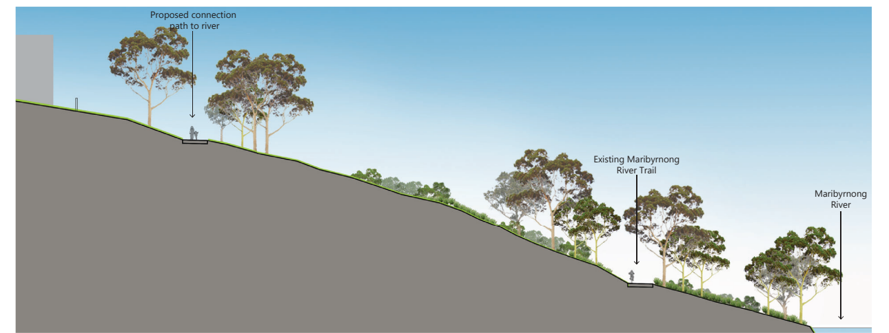
Section A-A
